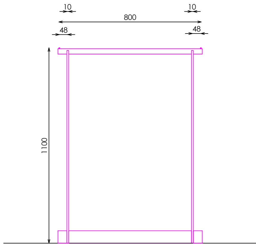
ALZADO
