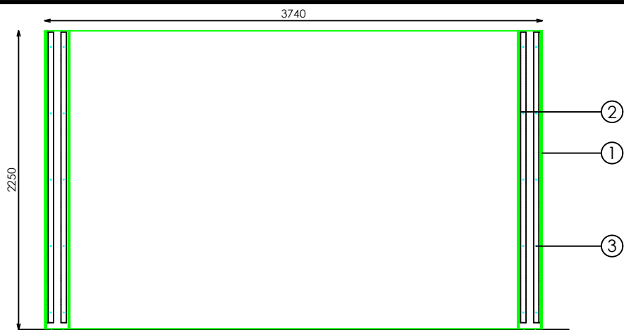
ALZADO POSTERIOR
