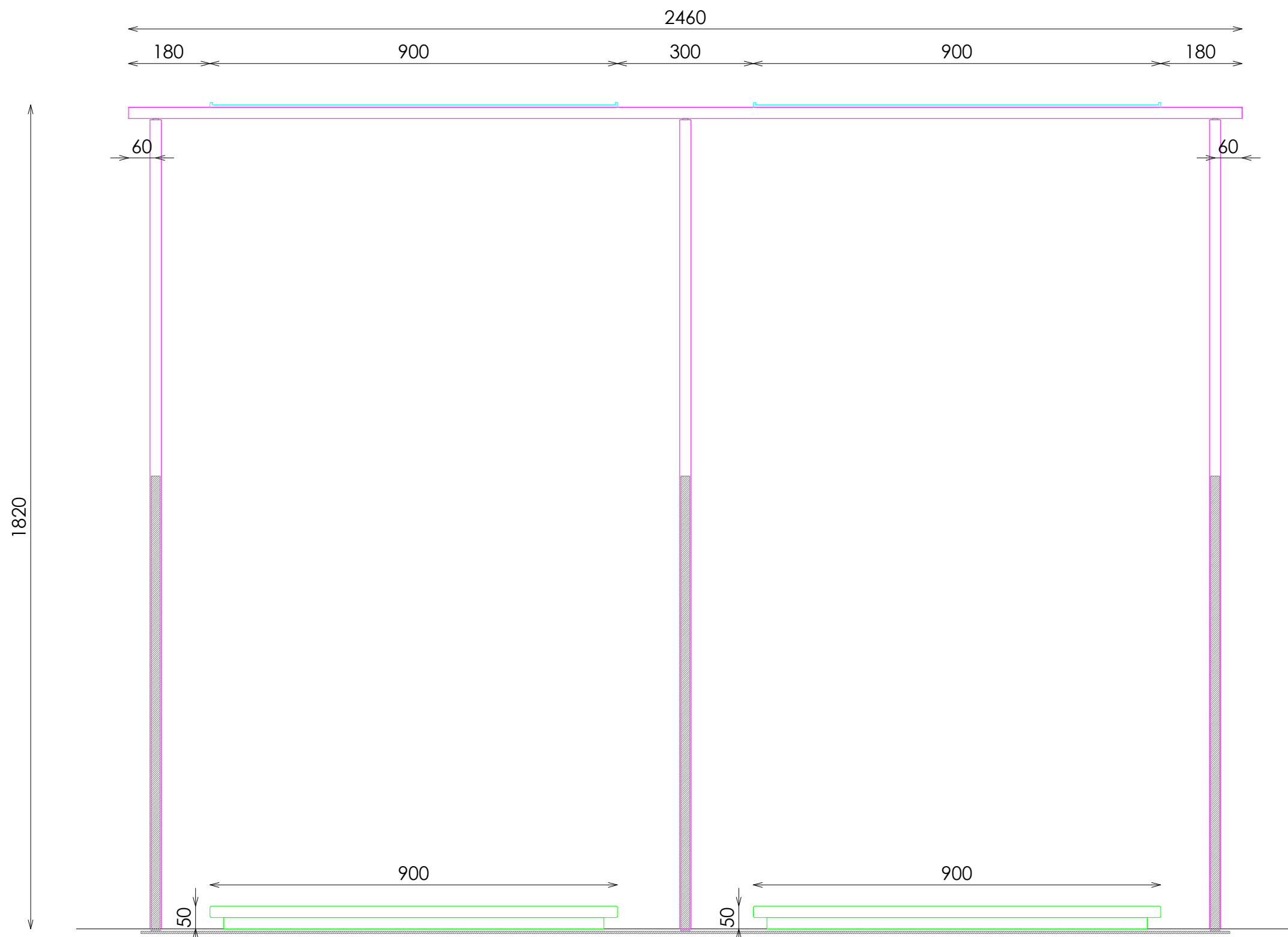
ALZADO
