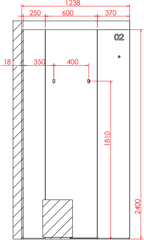
剖面 AG-AG
