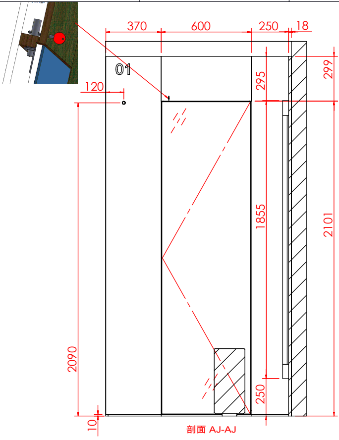
剖面 AJ-AJ
