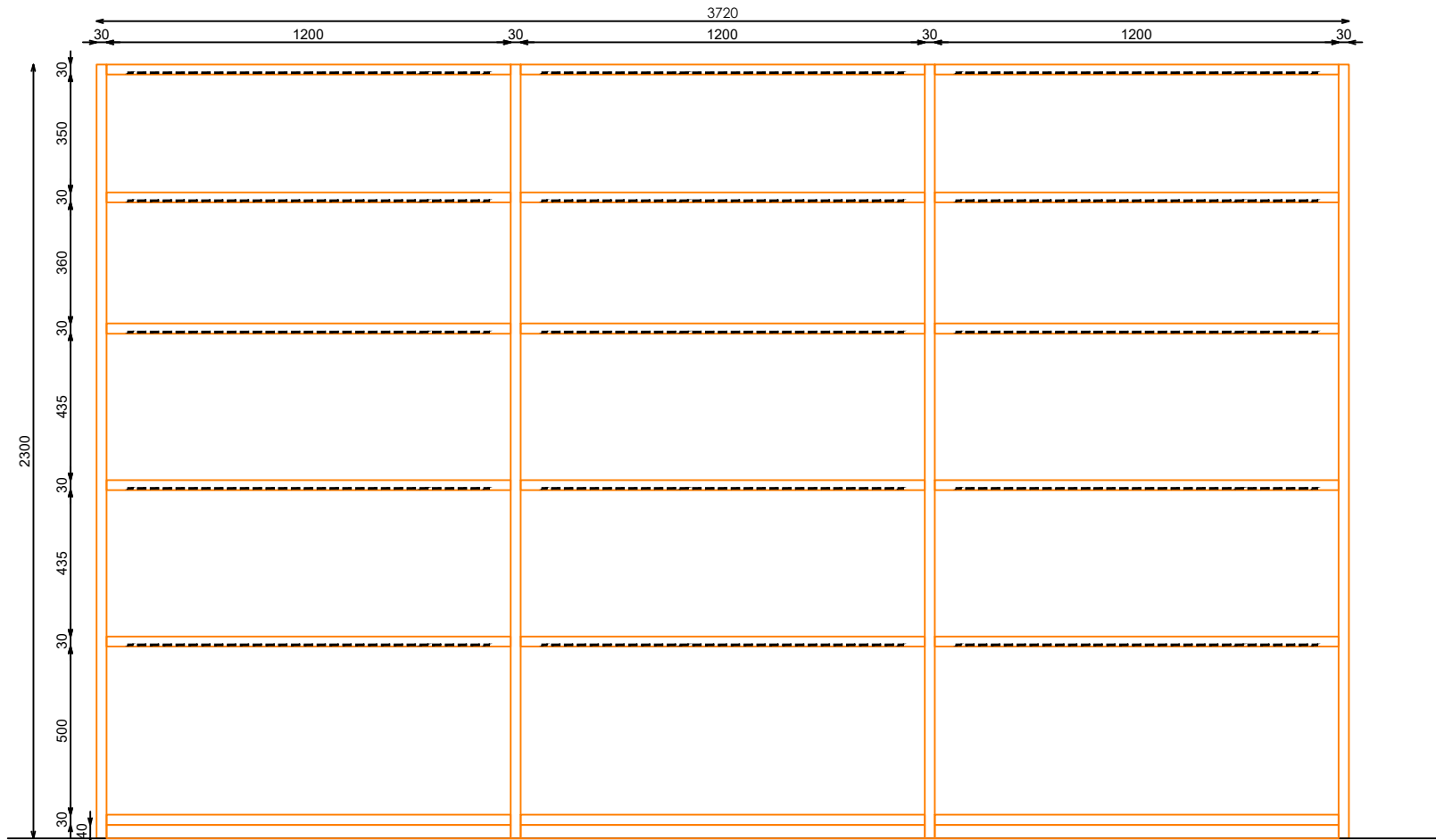
ALZADO
