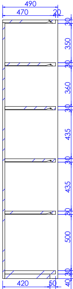
剖面 AG-AG
