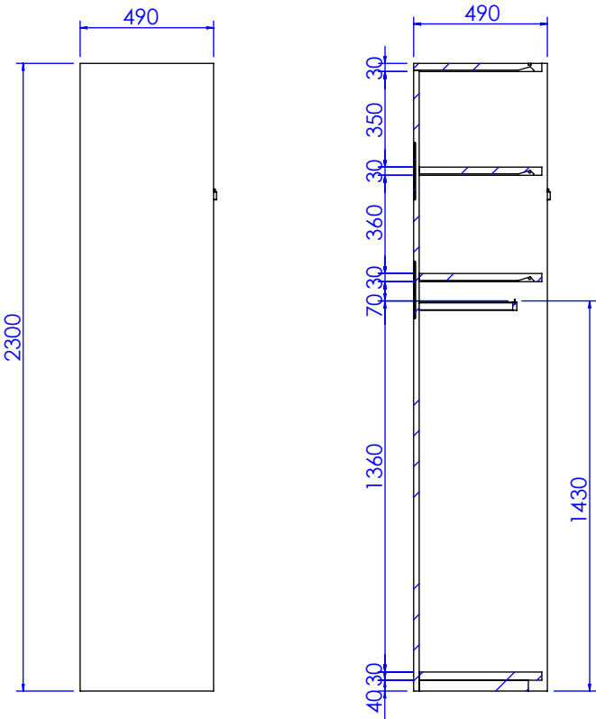
剖面 AG-AG
