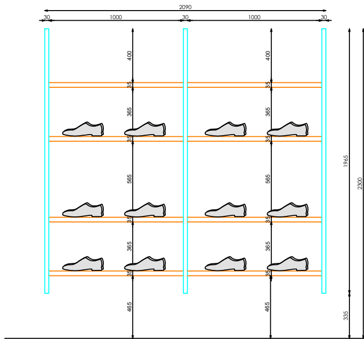
ALZADO FRONTAL
