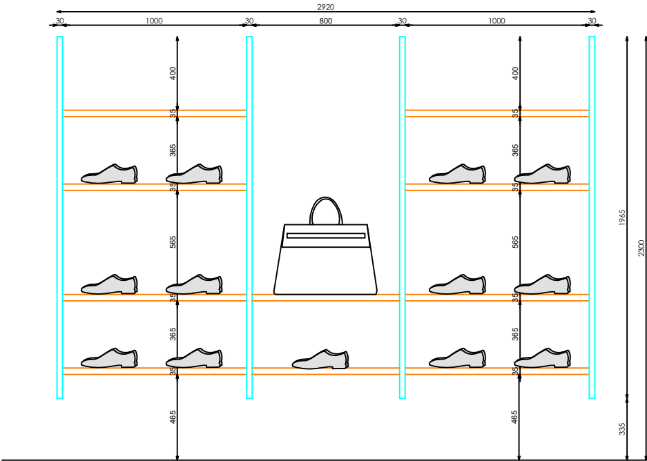
ALZADO FRONTAL
