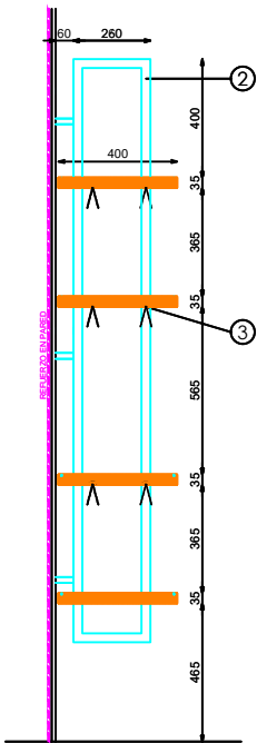
SECCION
