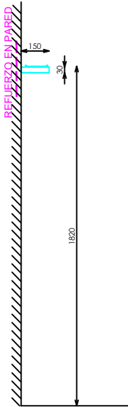
SECCION
