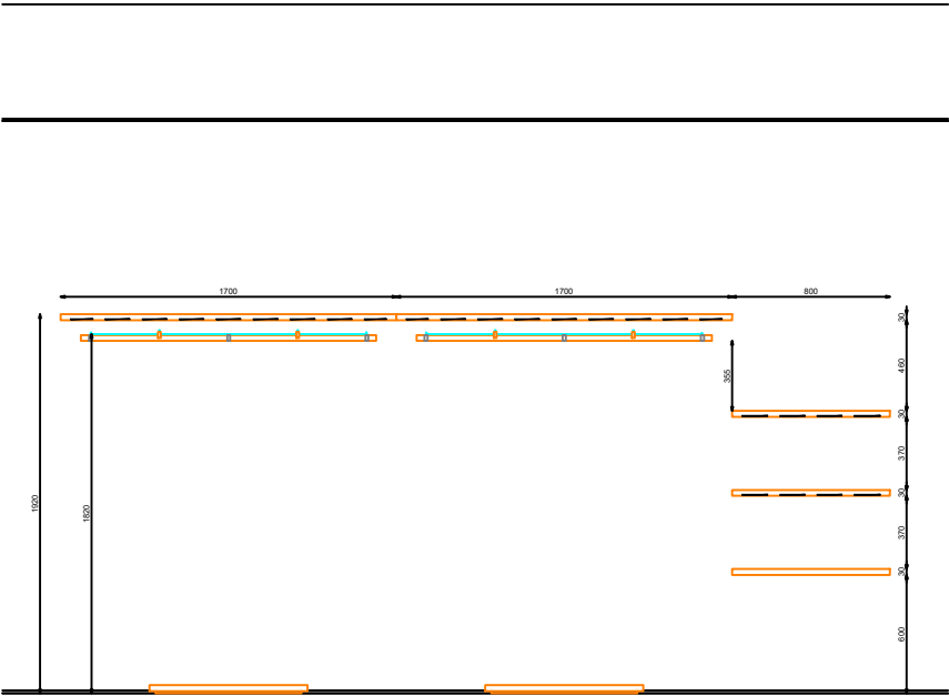
ALZADO FRONTAL
