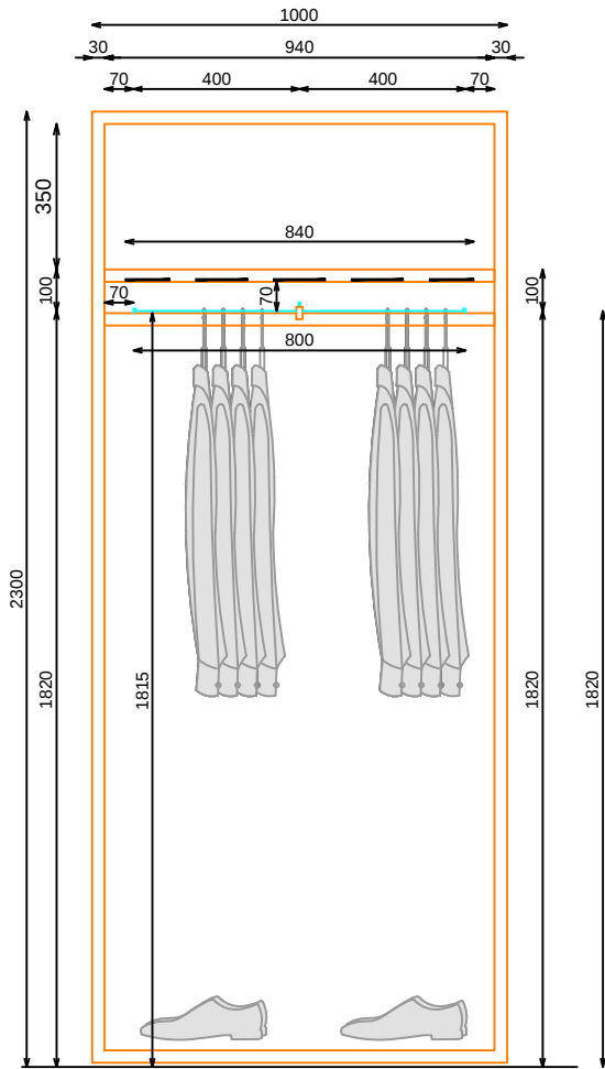
ALZADO
