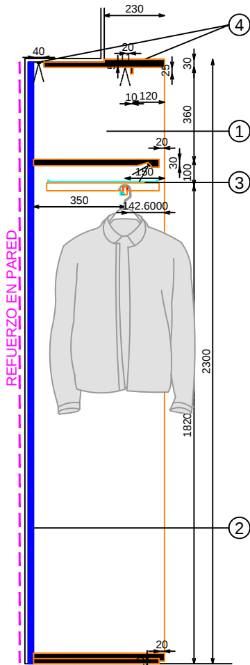
SECCION BARRA ALTA
