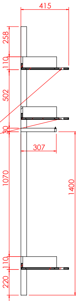
剖面 AH-AH
