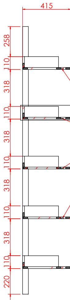
剖面 AG-AG
