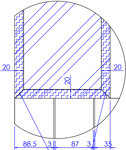
局部视图 K 比例 1 : 5
