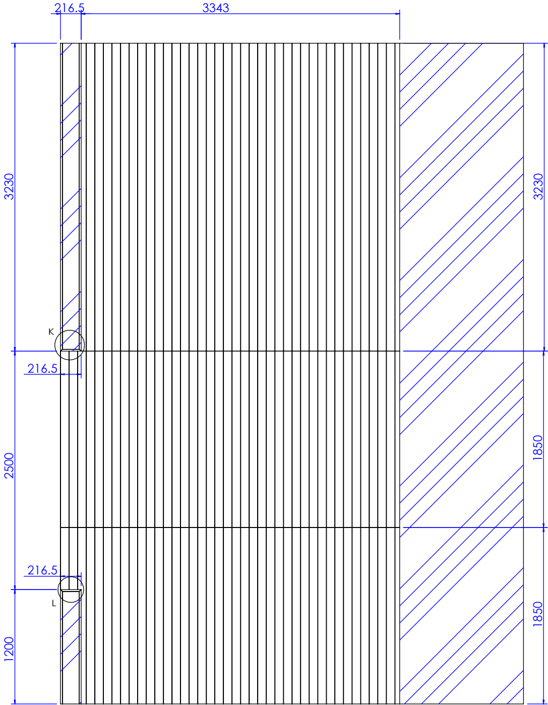
剖面 H-H
