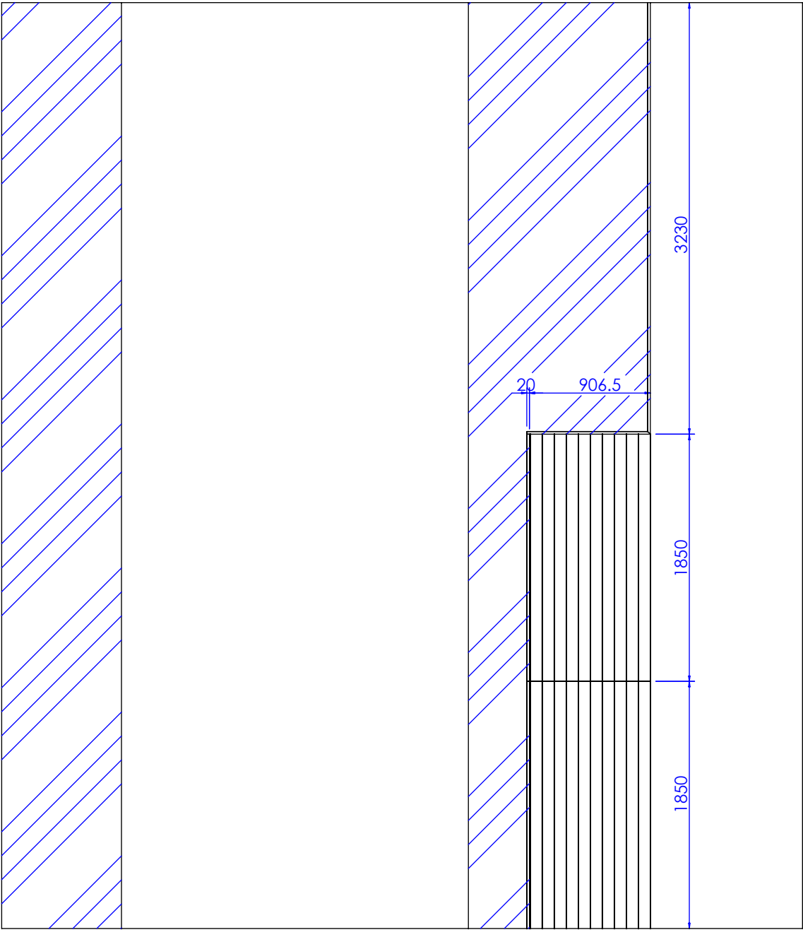
剖面 E-E
