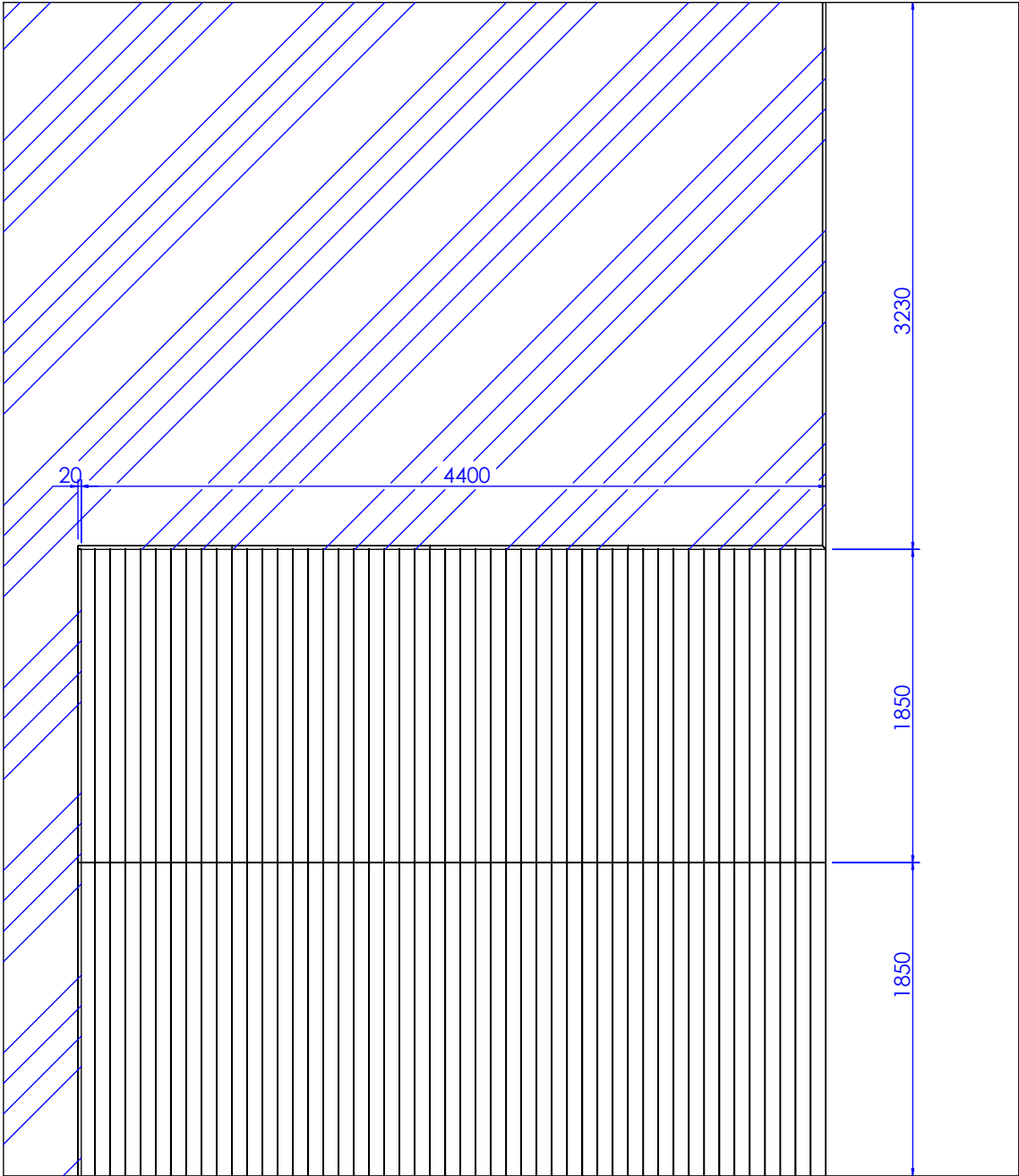
剖面 C-C
