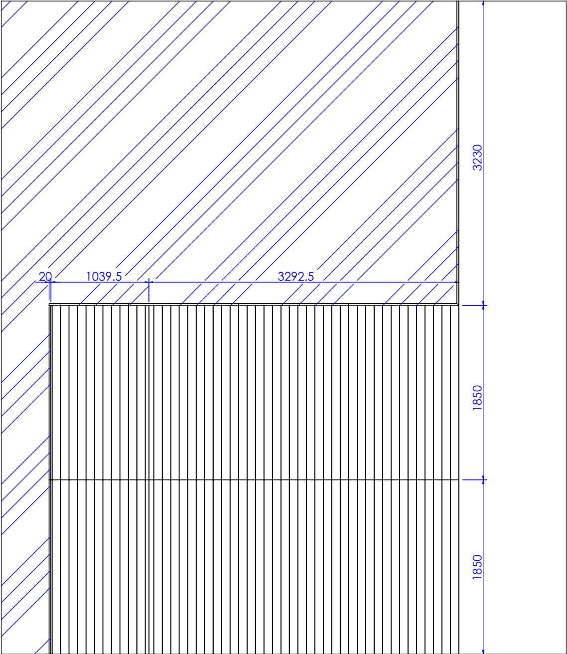
剖面 G-G
