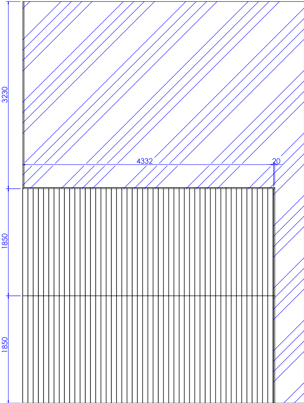
剖面 F-F
