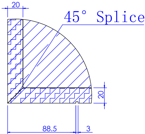
局部视图 I 比例 1 : 3
