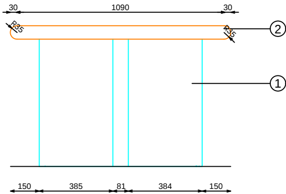
ALZADO LATERAL
