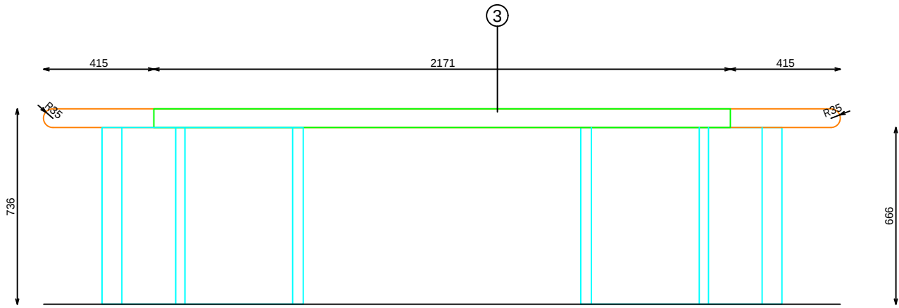
ALZADO FRONTAL
