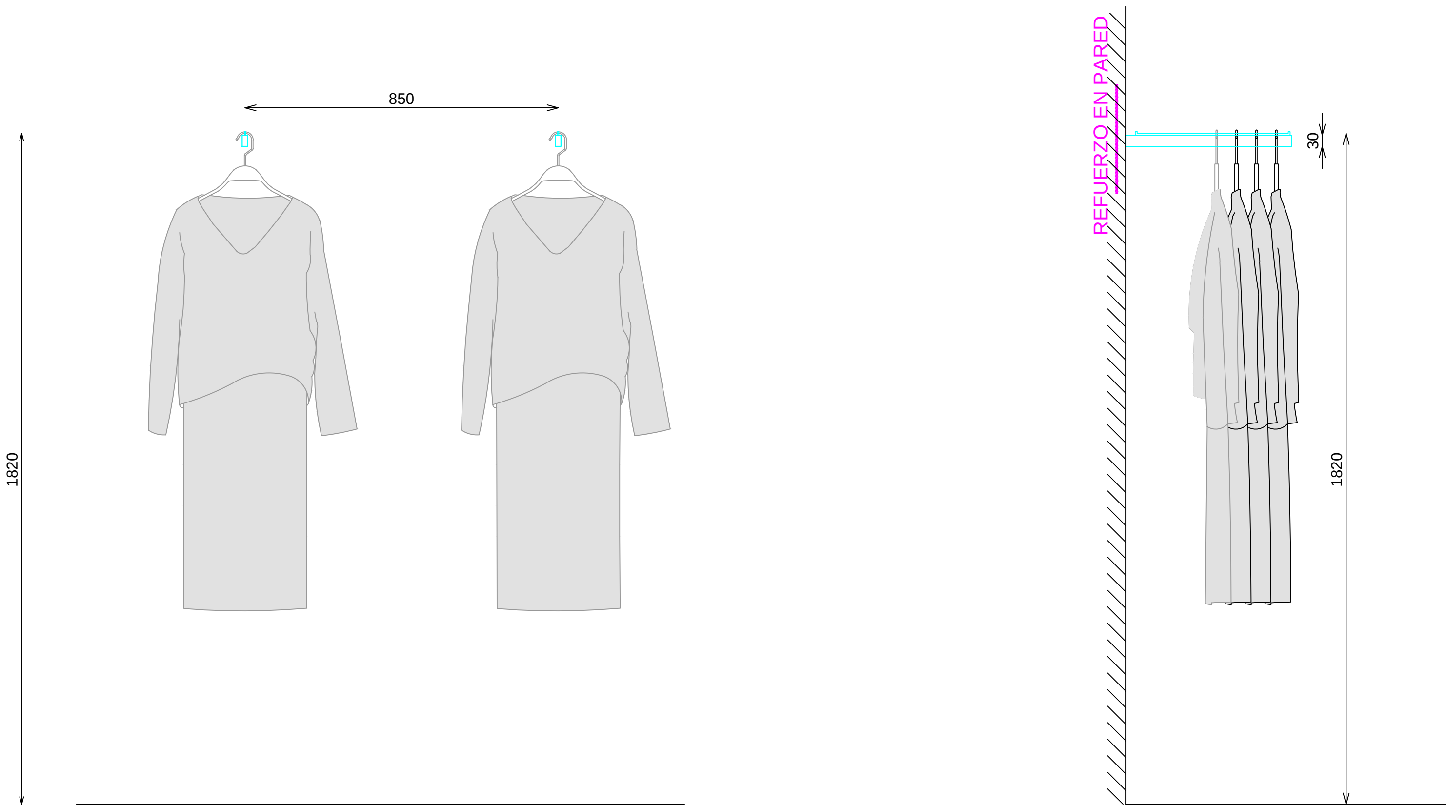
ALZADO FRONTAL
