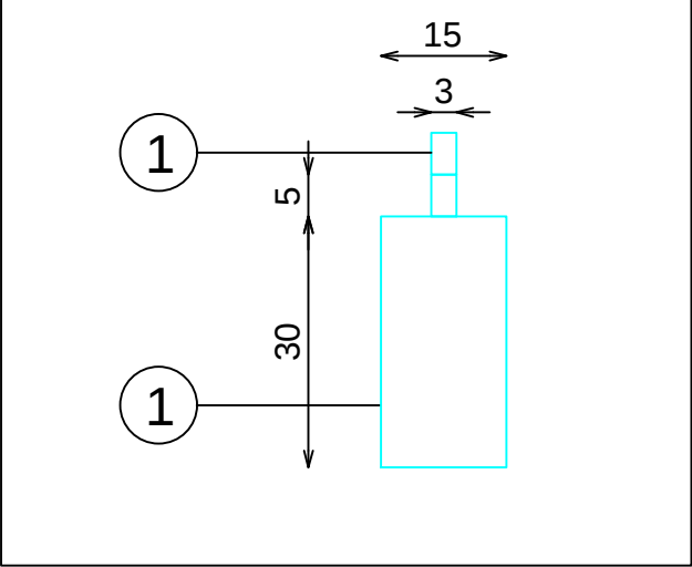
DETALLE BARRA
