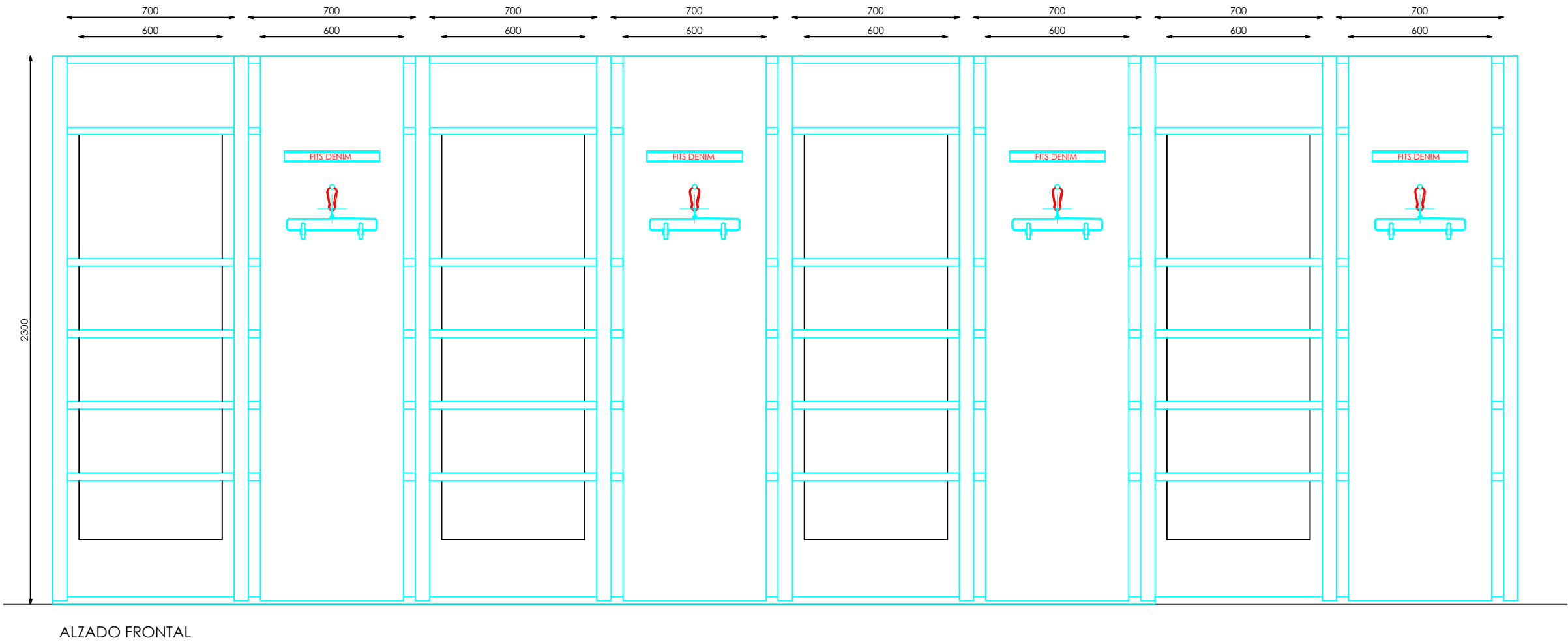
ALZADO FRONTAL
