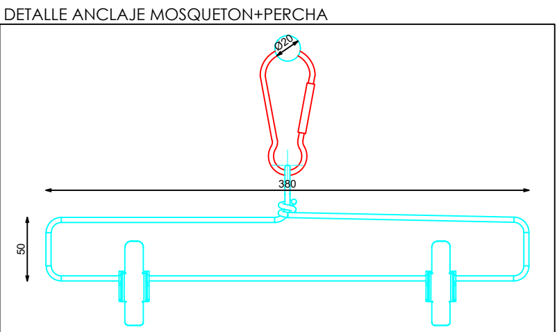
DETALLE PERCHA
