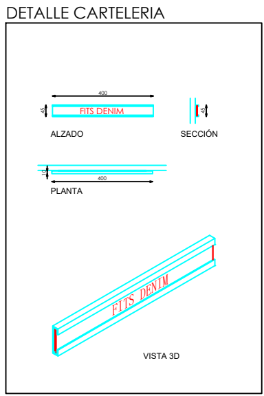
DETALLE CARTELERIA
