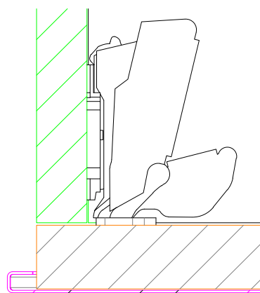
DETALLE C
