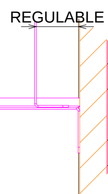
DETALLE B
