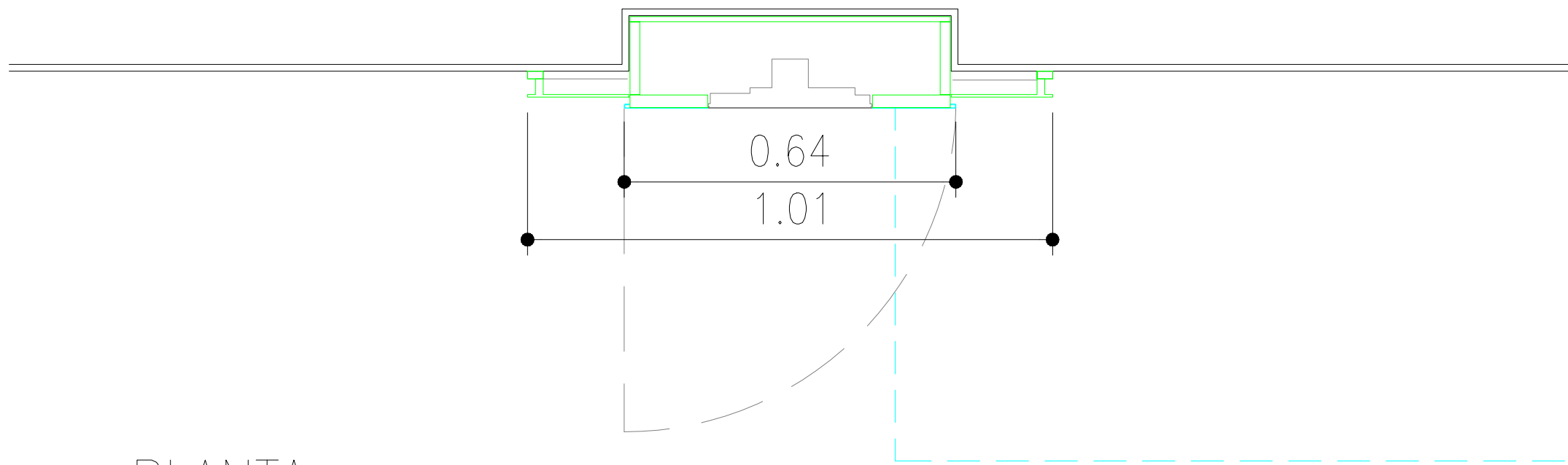
PLANTA
