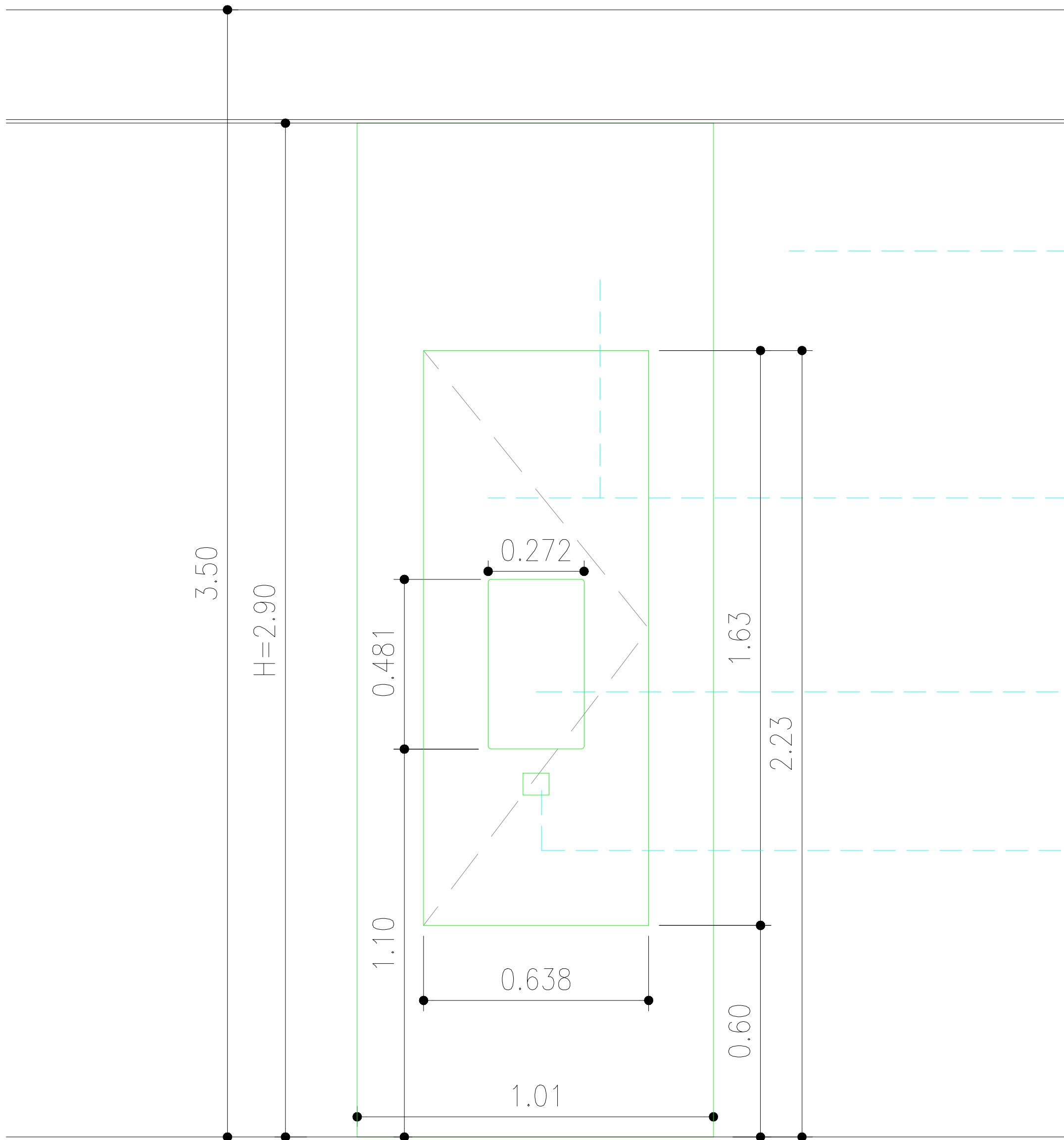
ALZADO
