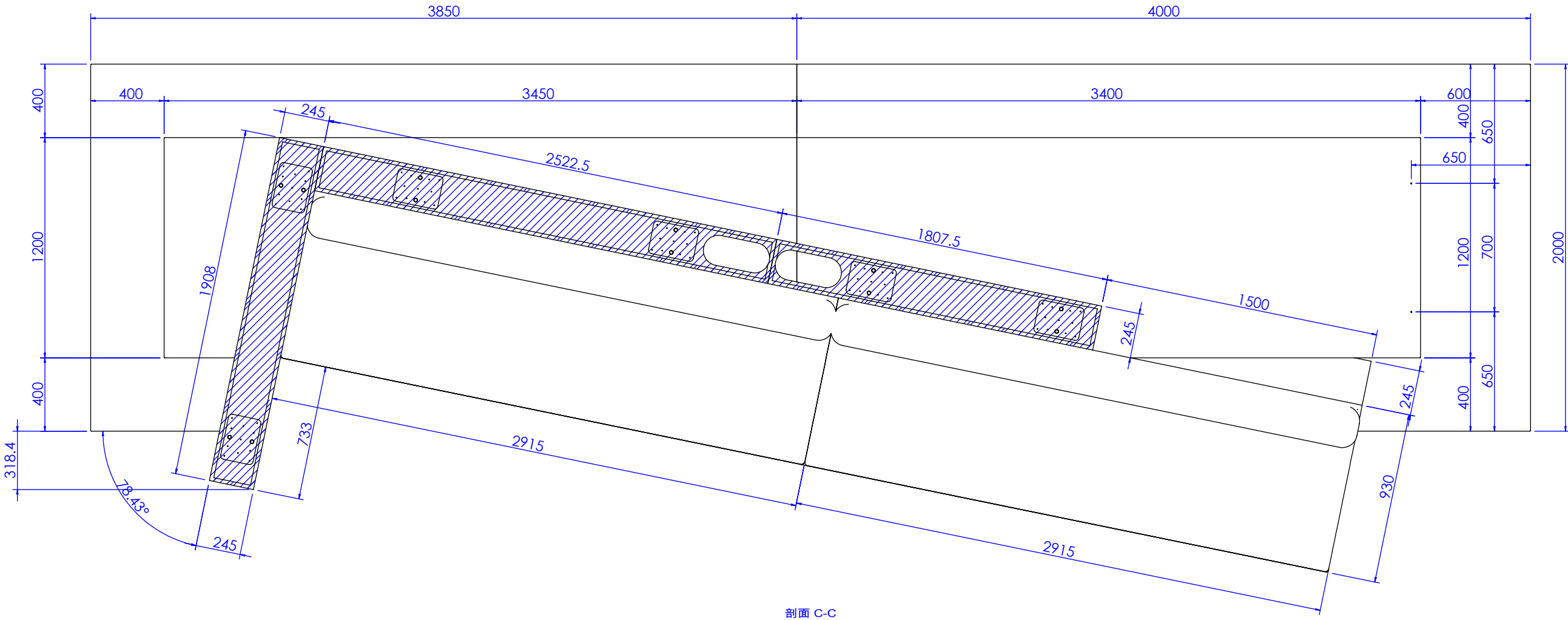
剖面 C-C
