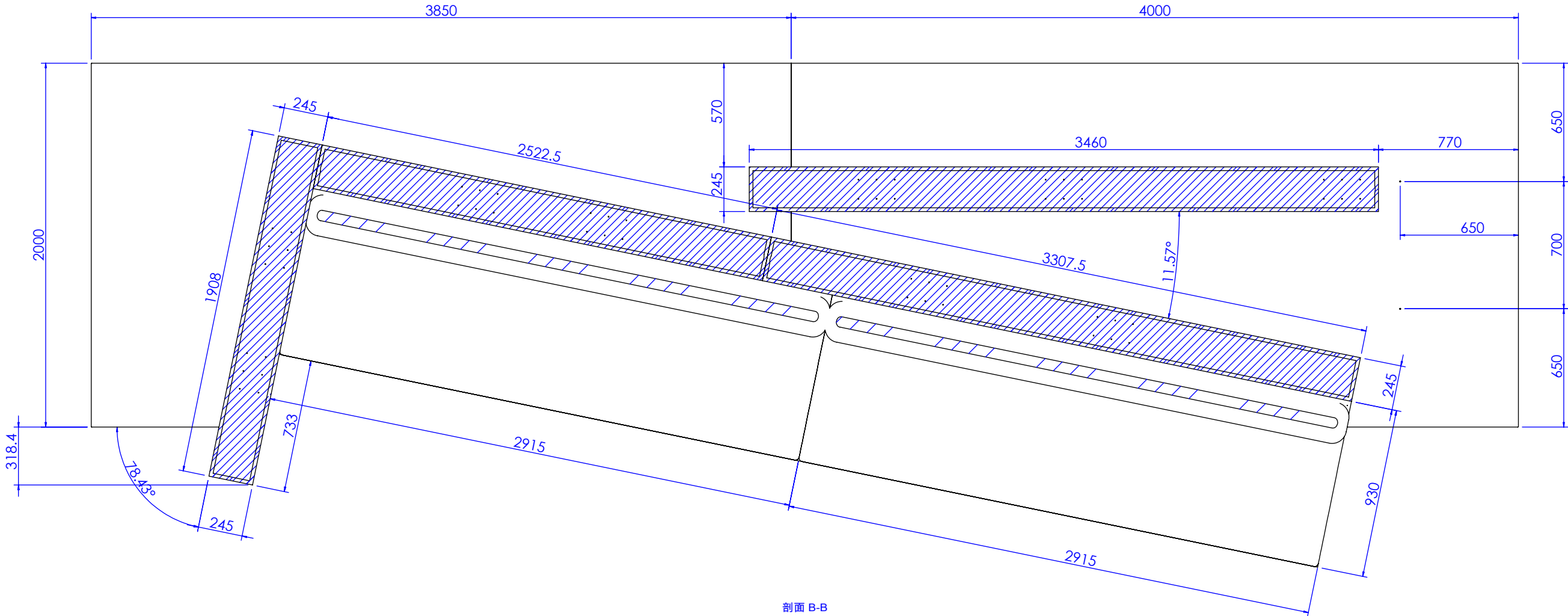
剖面 B-B
