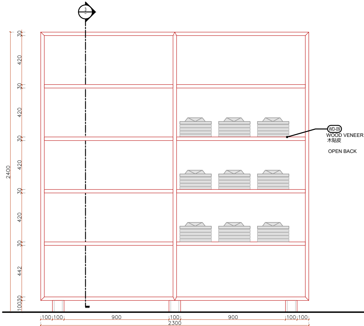
2 正立面 1:10 FRONT ELEVATION
