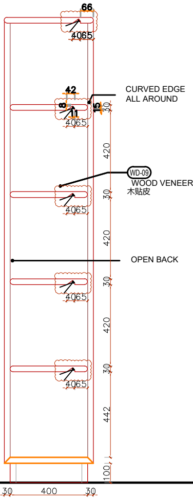
3 正立面 1:10 SIDE ELEVATION
