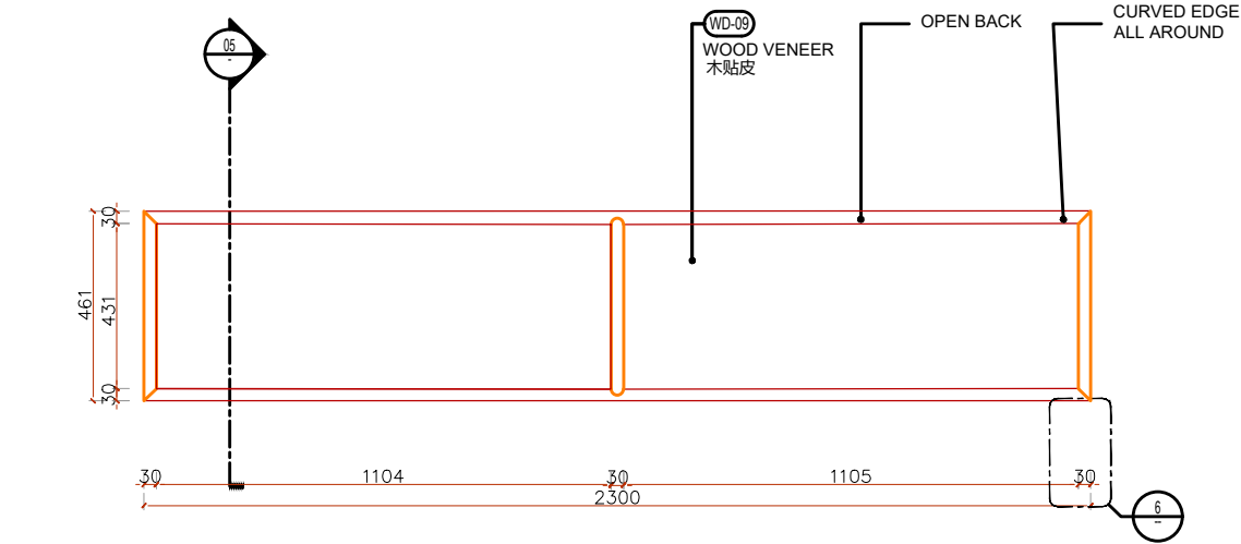
1 正立面 1:10 PLAN
