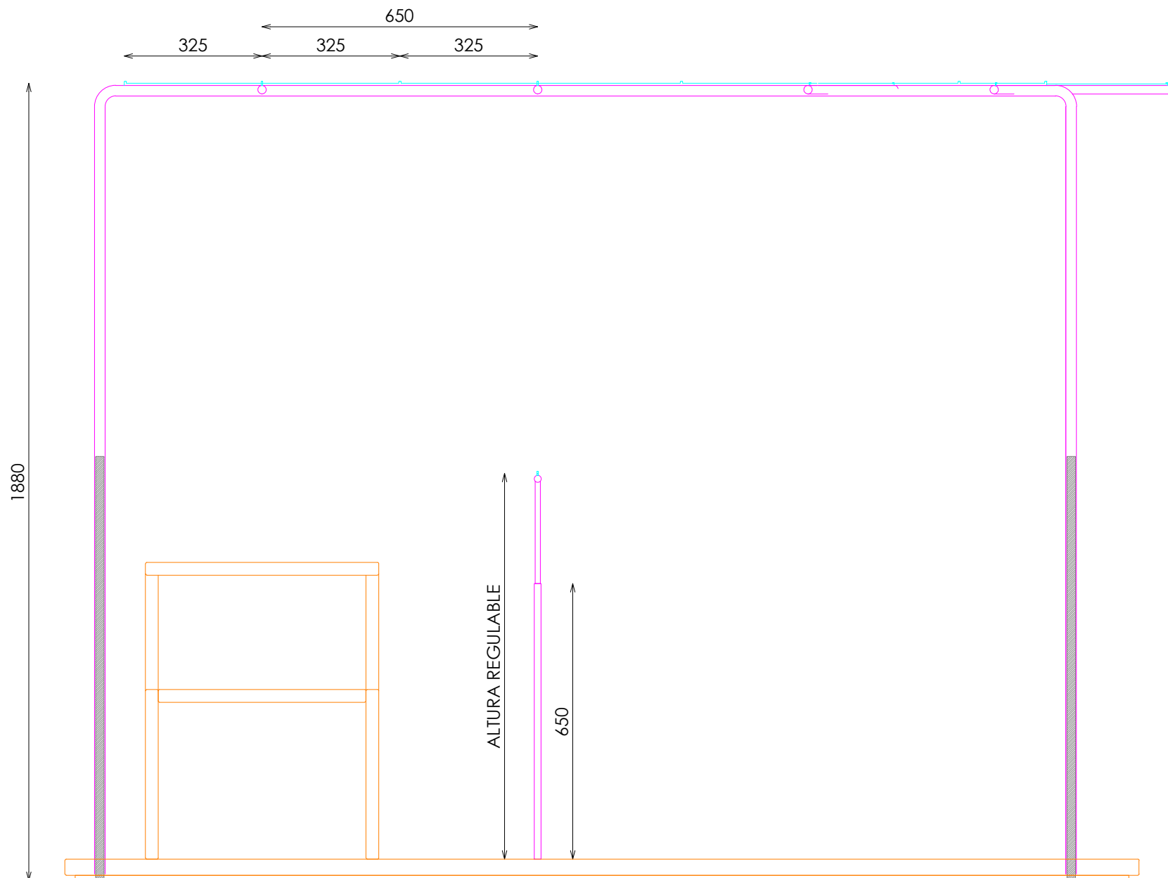
ALZADO FRONTAL
