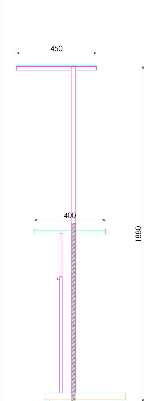
ALZADO LATERAL
