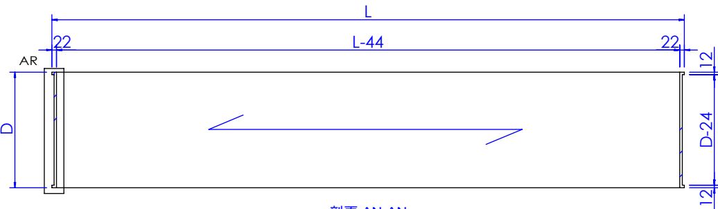
剖面 AN-AN
