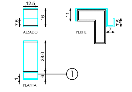
DOTACION CUELGA FRONTAL
