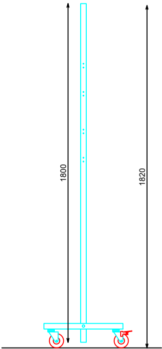
ALZADO LATERAL
