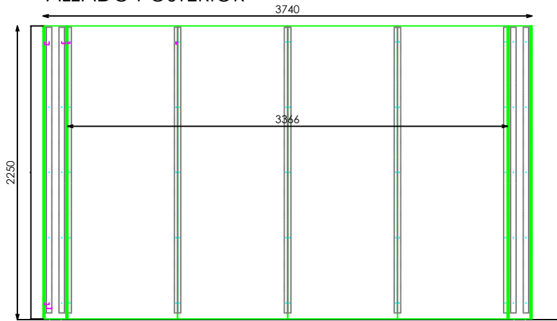
ALZADO FRONTAL
