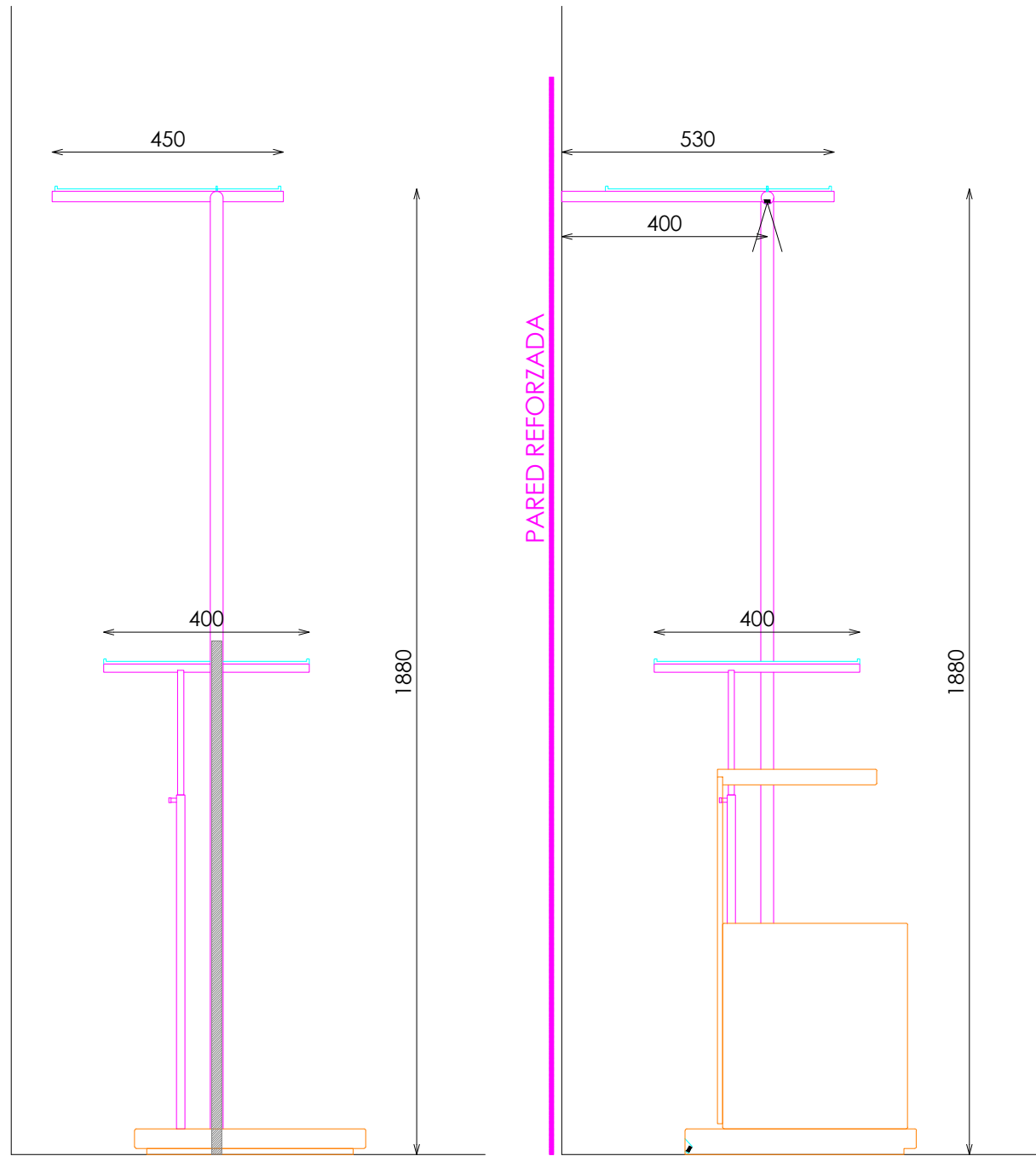
ALZADO LATERAL
