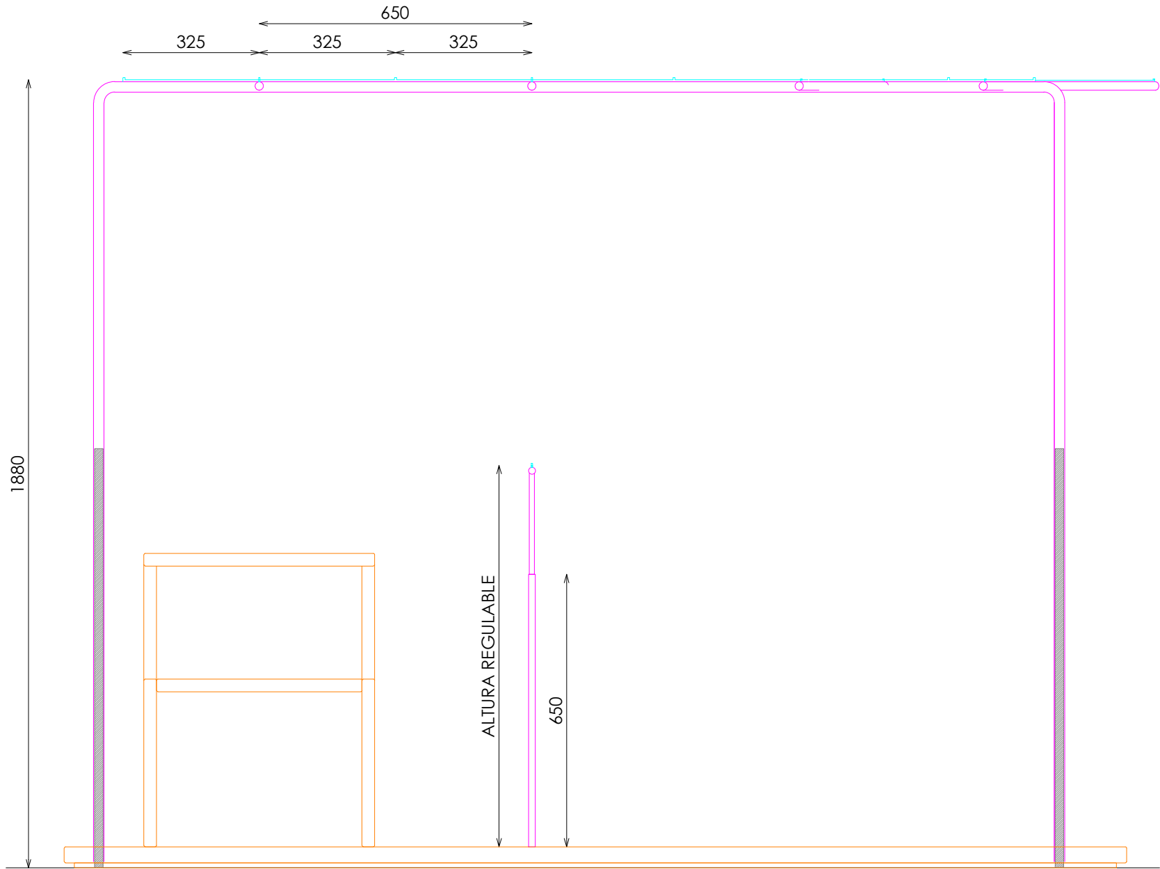
ALZADO FRONTAL
