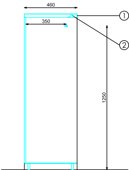
SECCION
