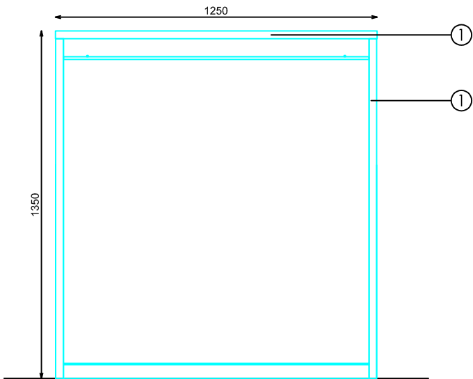
ALZADO FRONTAL
