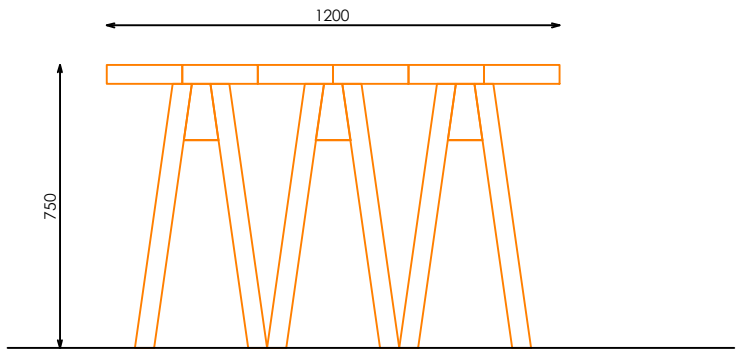
PERFIL
