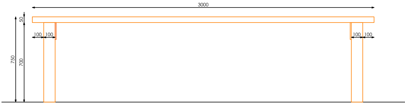
ALZADO FRONTAL
