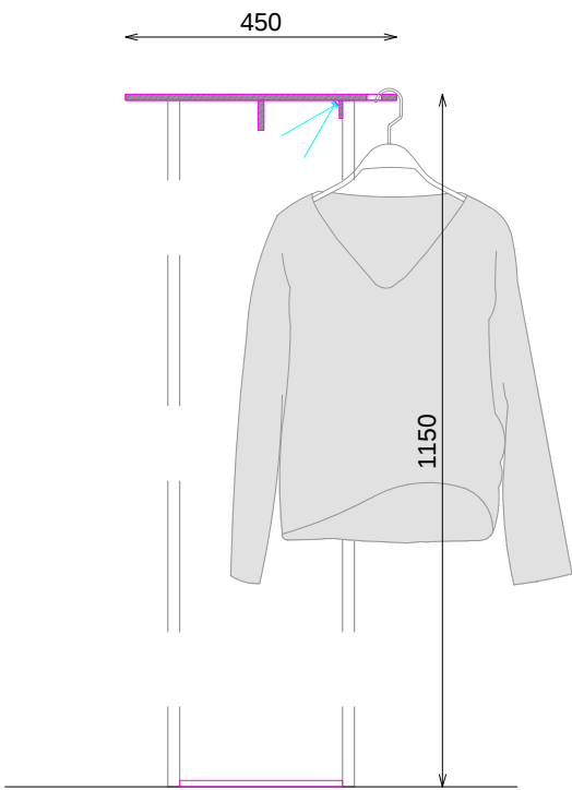
SECCIÓN CUELGA
