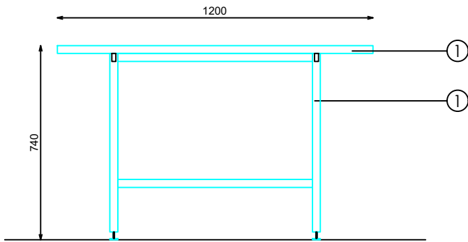
ALZADO LATERAL
