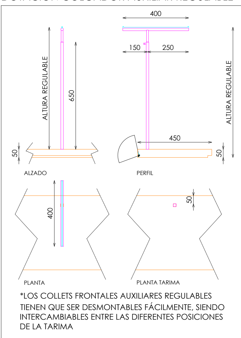
DETALLE A
