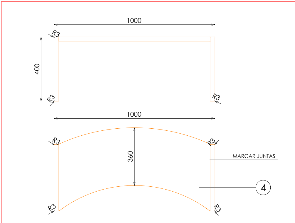
BANCO CURVO 100. SOLO BAJO PETICION DPTO. MERCHANDISING
