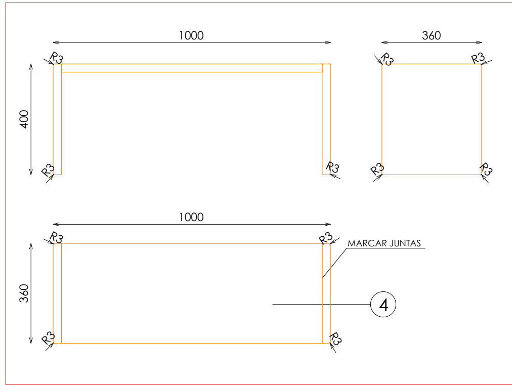
BANCO RECTO 100. SOLO BAJO PETICION DPTO. MERCHANDISING
