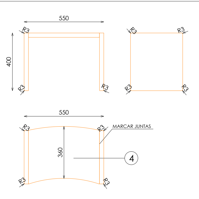
BANCO CURVO 55
