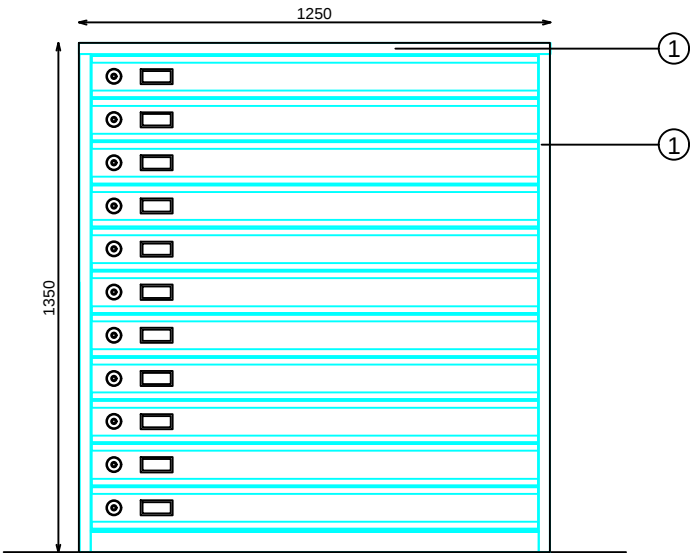
ALZADO FRONTAL
