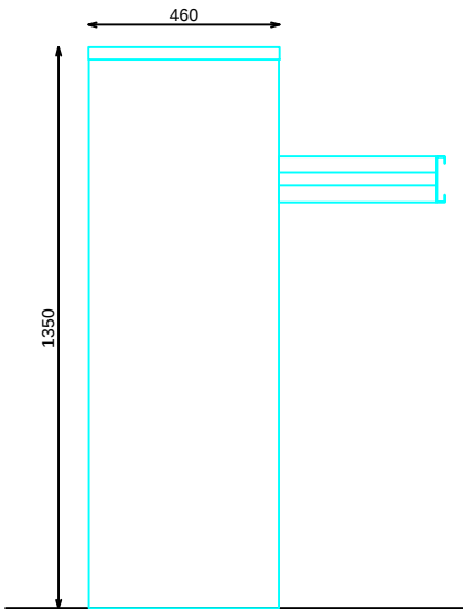
ALZADO LATERAL
