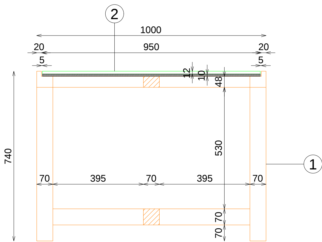
SECCION
