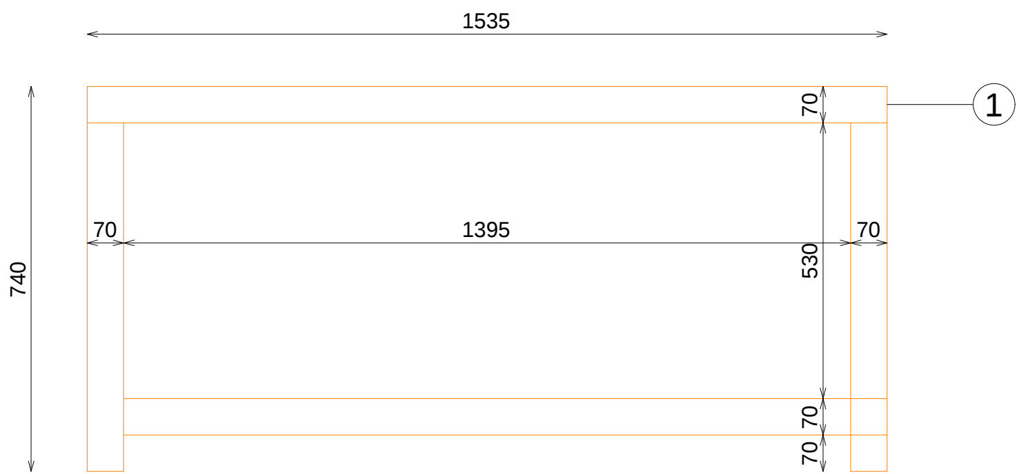
ALZADO FRONTAL
