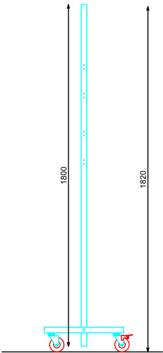
ALZADO LATERAL
