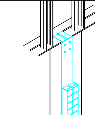
DETALLE ANCLAJE
