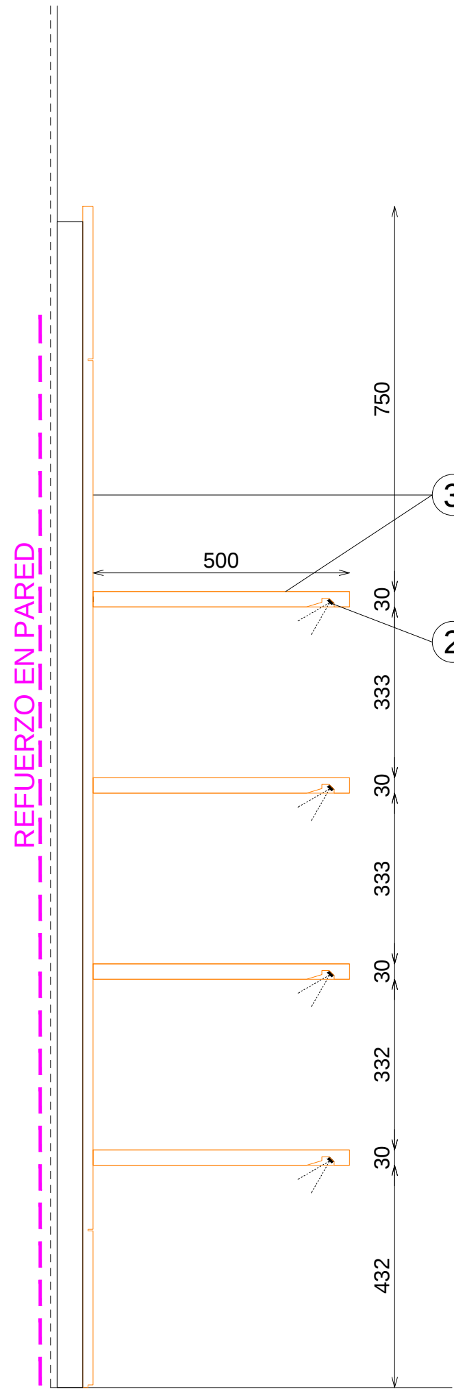
SECCION BALDAS
