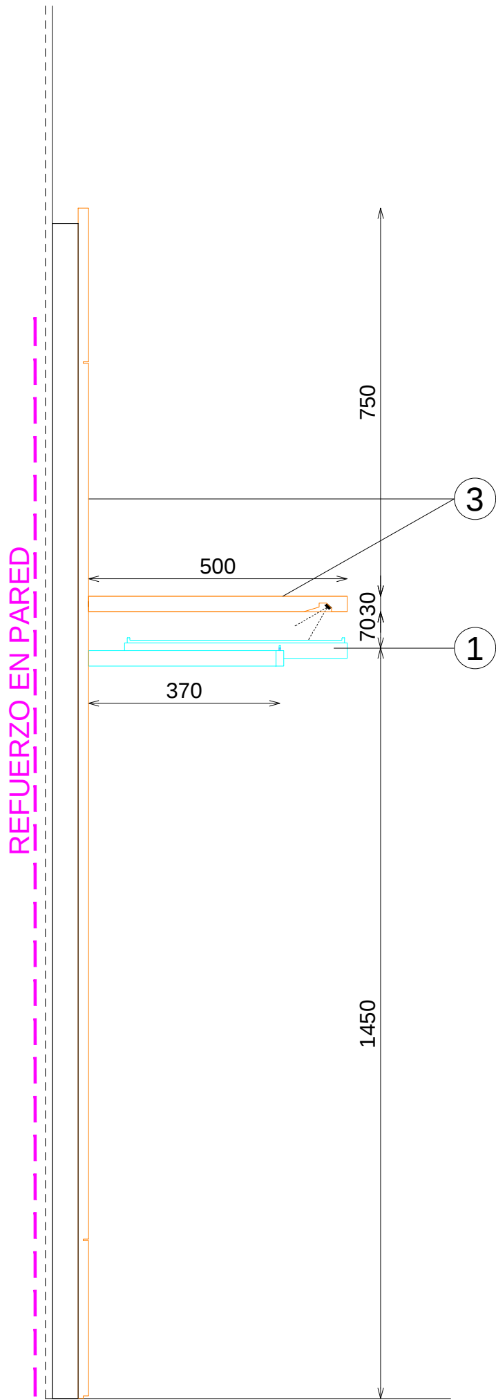
SECCION BARRA
