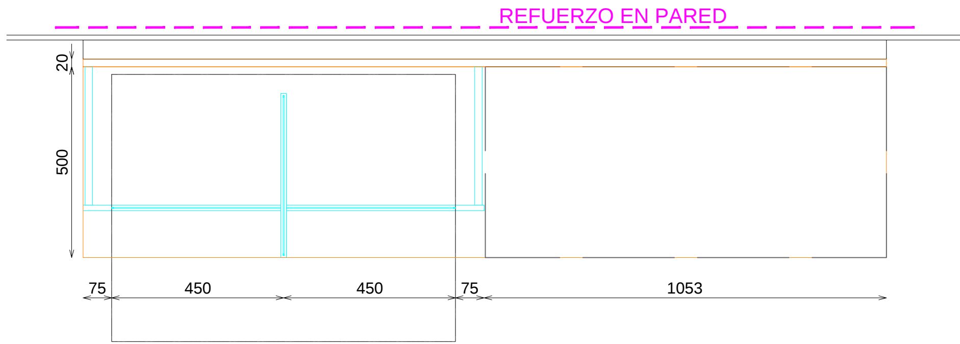
PLANTA
