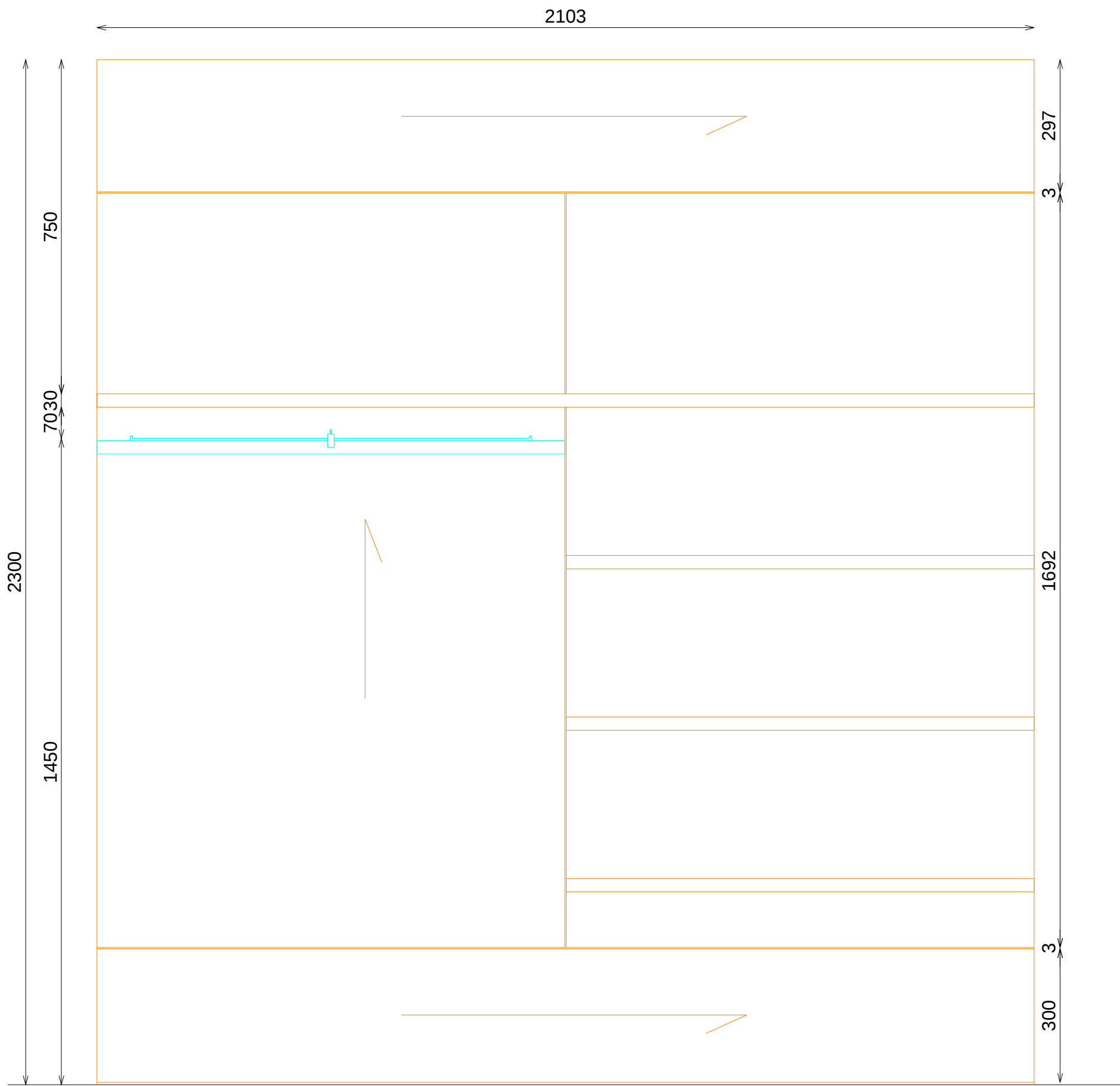
ALZADO
