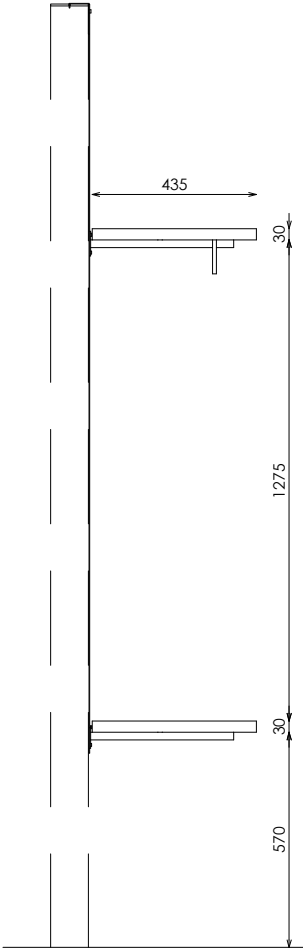
PERFIL
