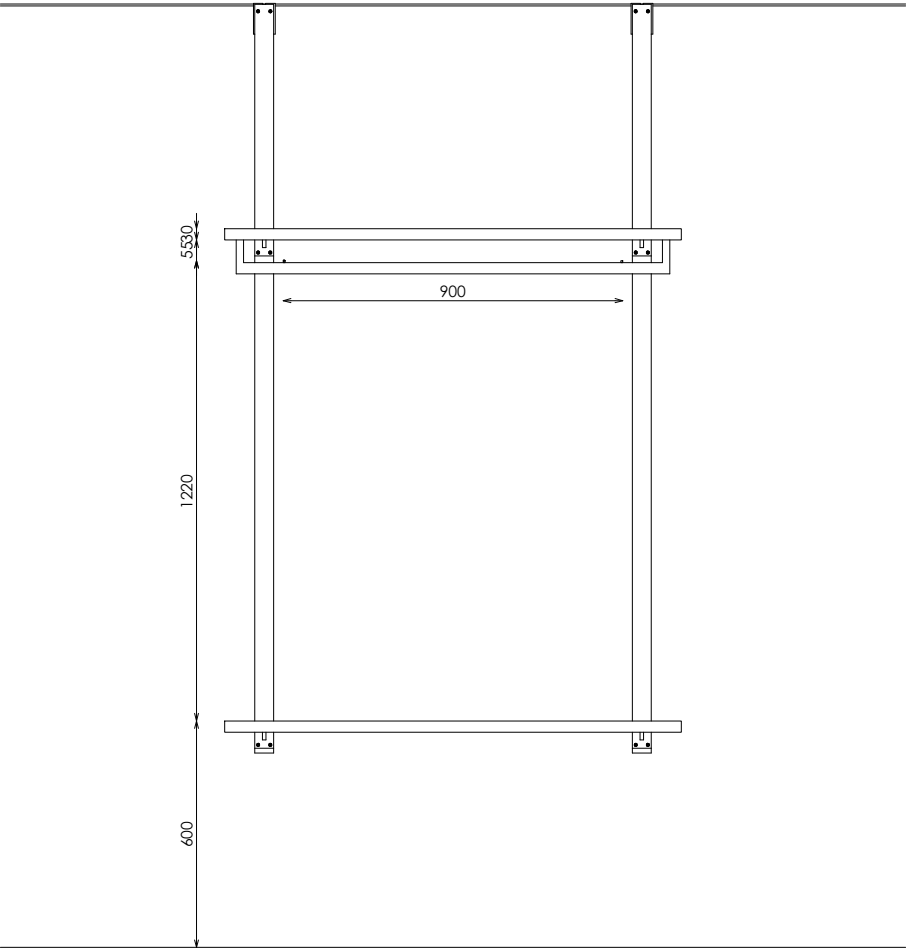
ALZADO
