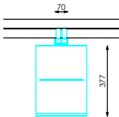
PLANTA
