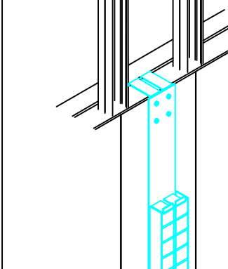
DETALLE ANCLAJE
