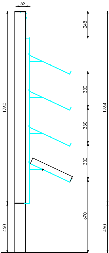
PERFIL
