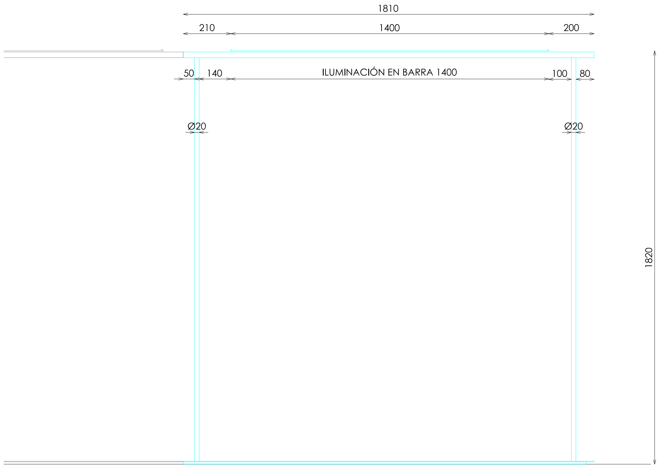
ALZADO FRONTAL
