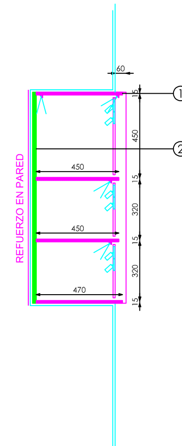
SECCION
