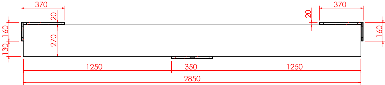
剖面 AG-AG
