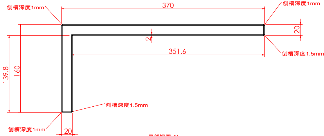
局部视图 AI 比例 1 : 4
