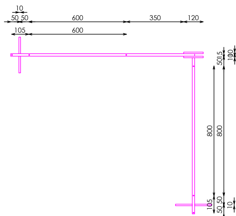
PLANTA
