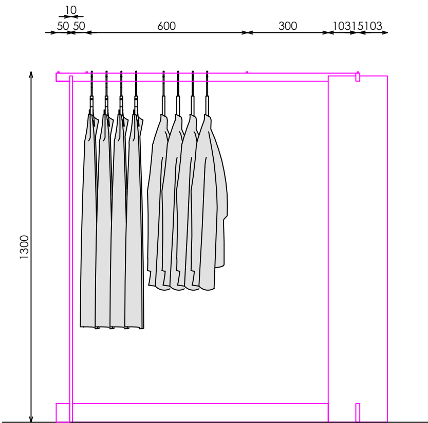
ALZADO
