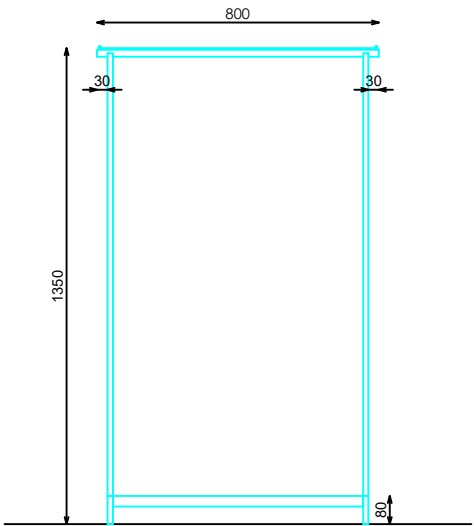
ALZADO
