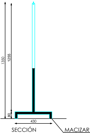
SECCIÓN
