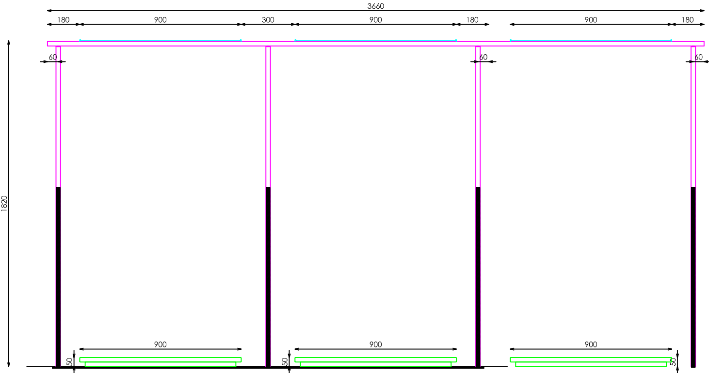
ALZADO
