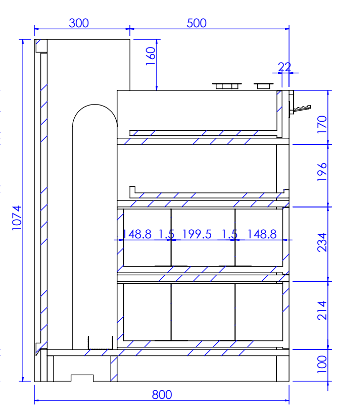
剖面 B-B
