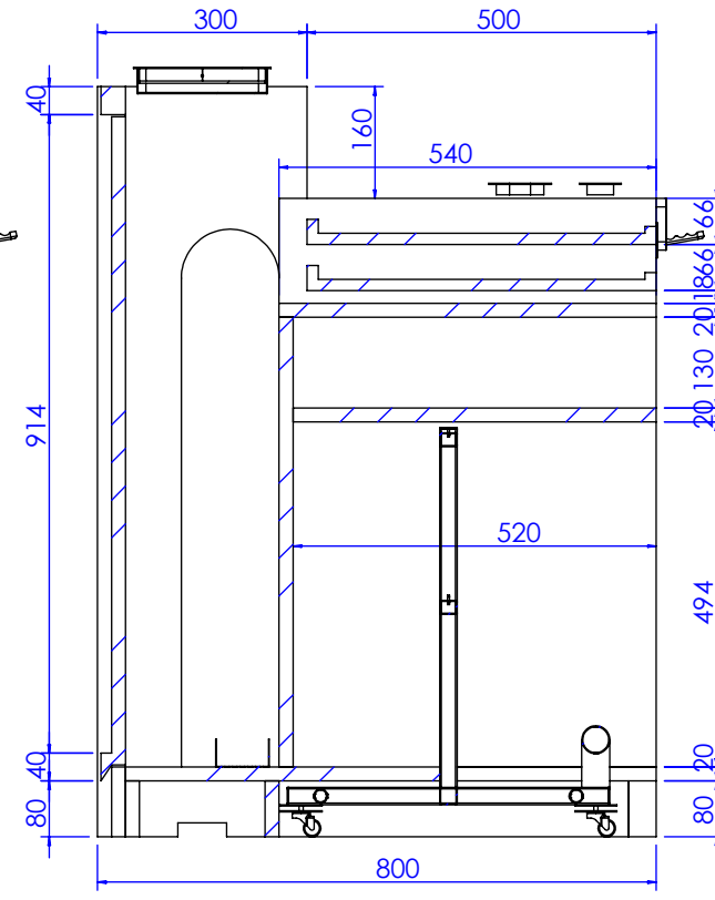
剖面 A-A
