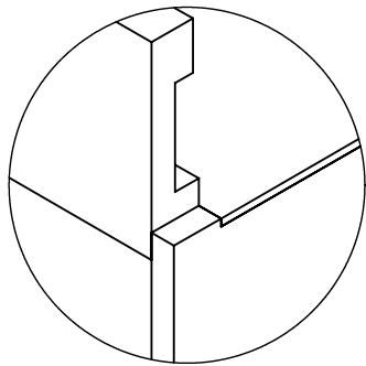
局部视图 Q 比例 1 : 5
