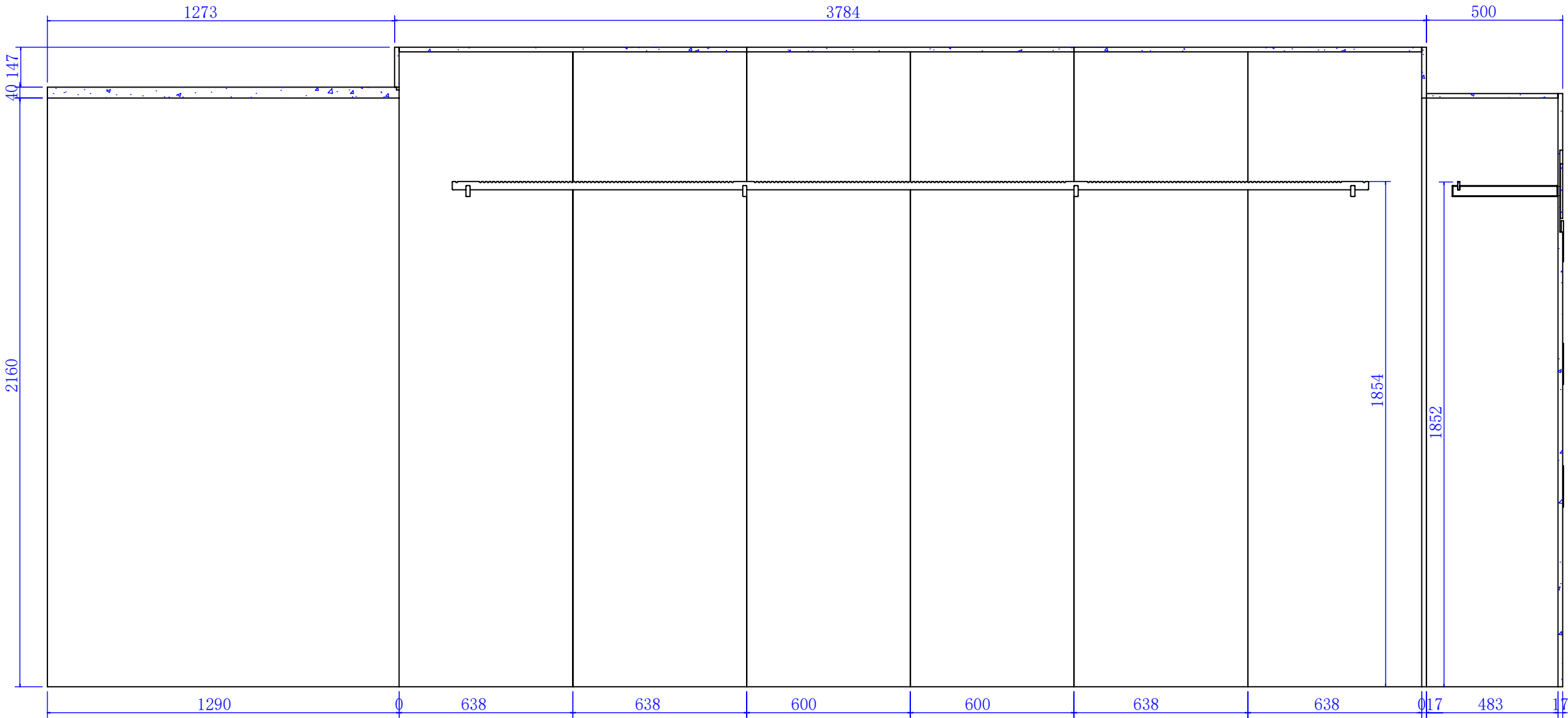
剖面 C-C
