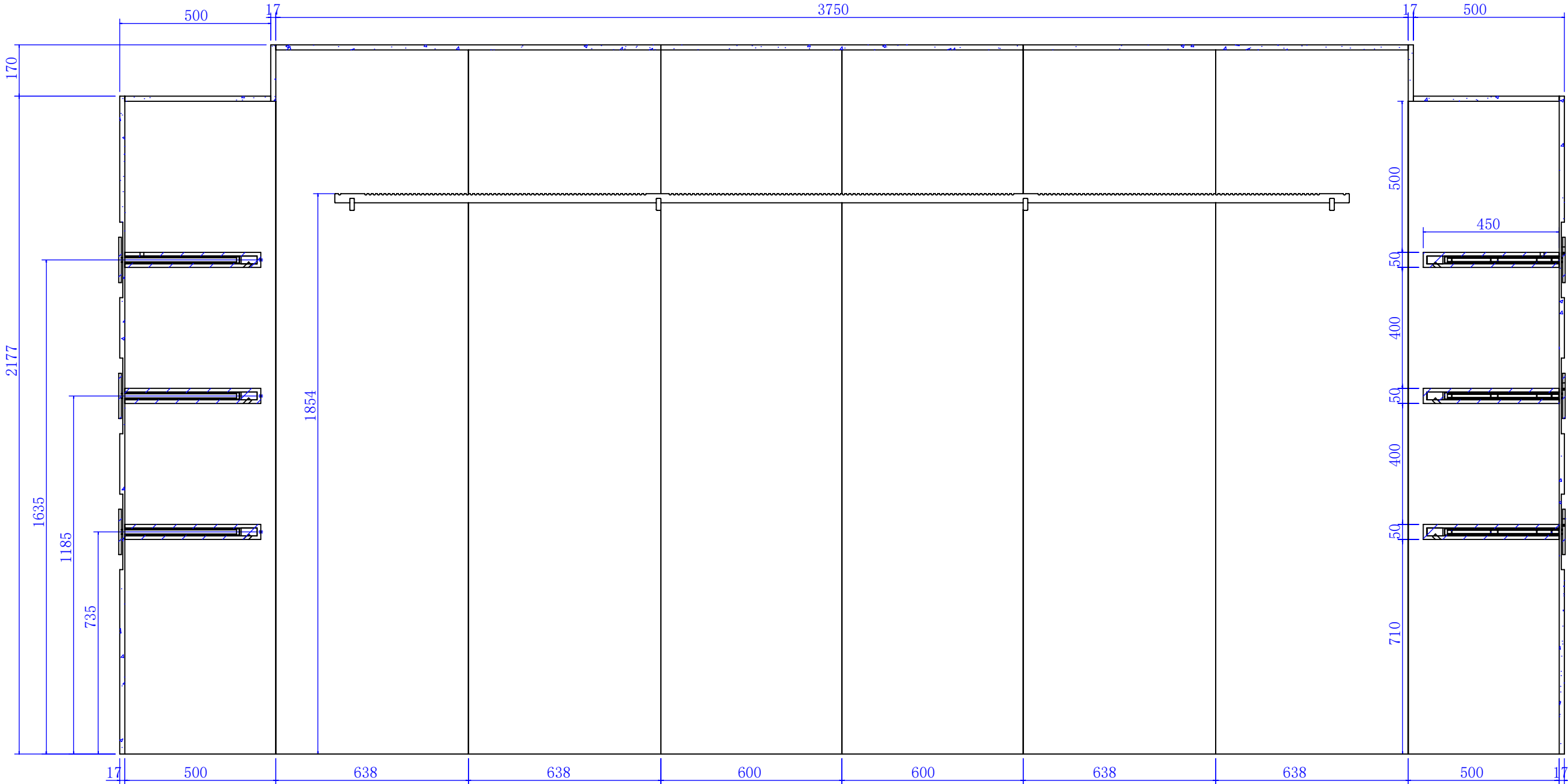
剖面 B-B
