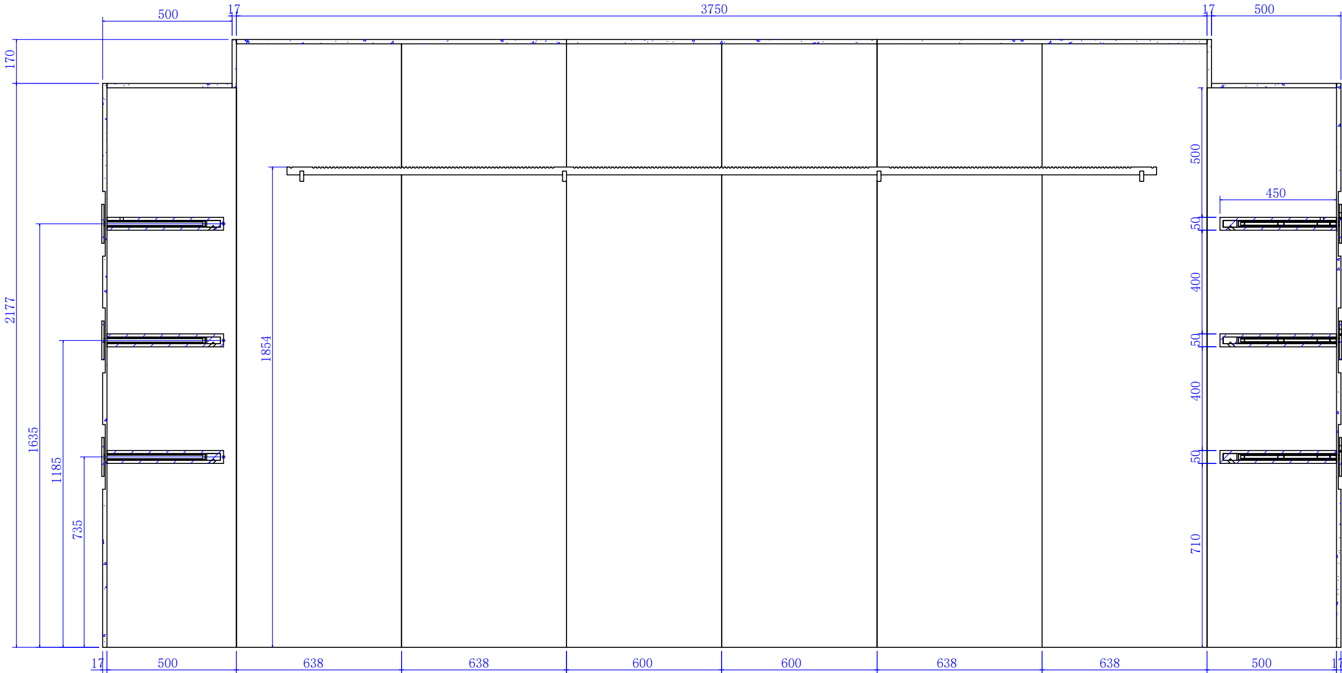
剖面 B-B
