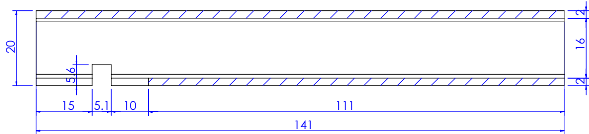
剖面 AS-AS
