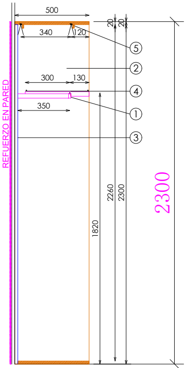
SECCIÓN
