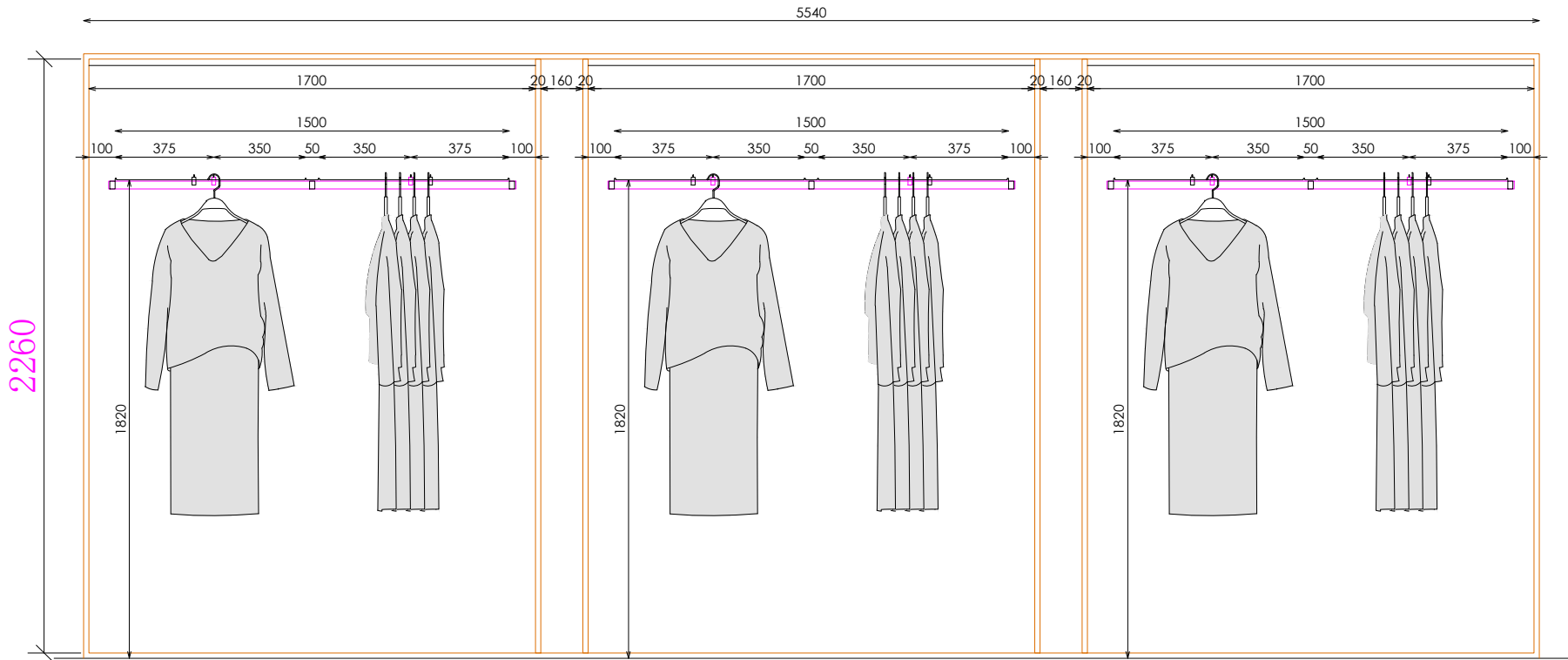
ALZADO
