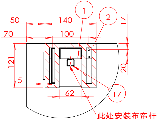
局部视图 D
