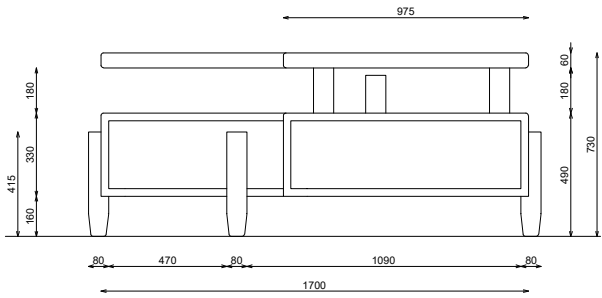
ALZADO LATERAL IZQUIERDDO
